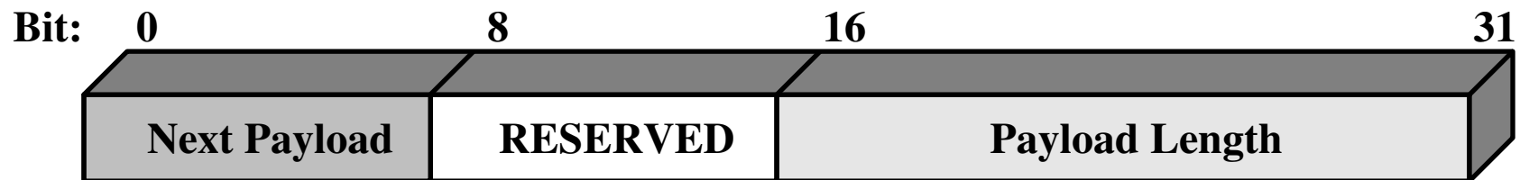
(b) Generic Payload Header
